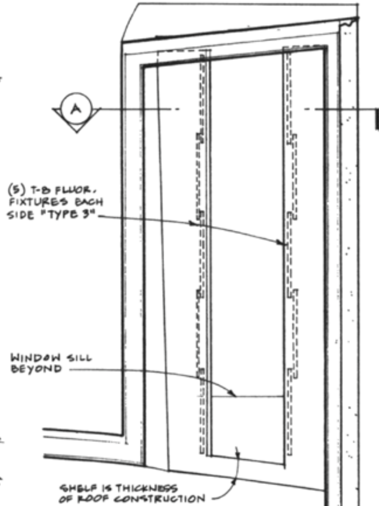
B ELEVATION \frac{1}{4}'' = 1'-0''
