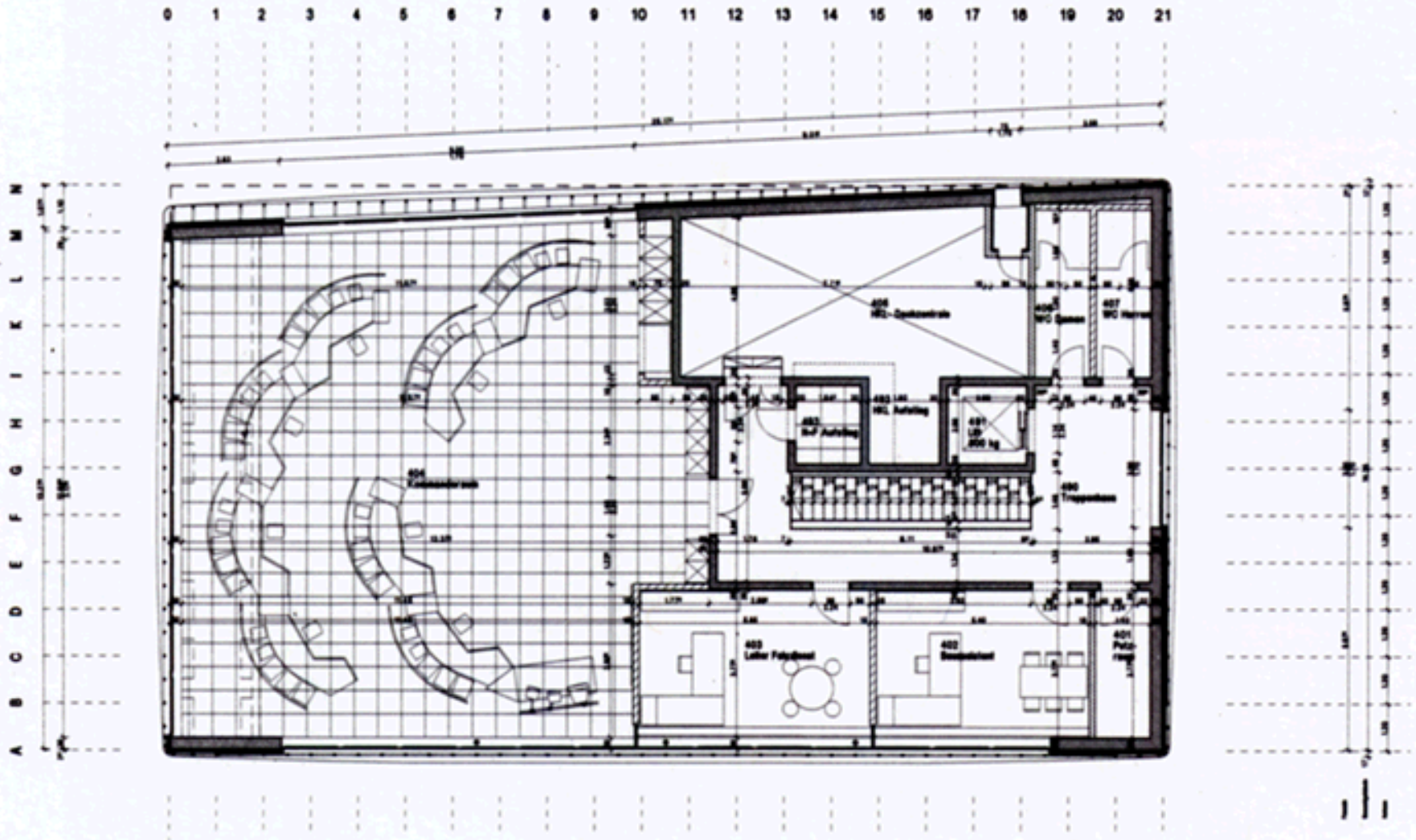
Planta cuarta / Fourth floor plan
