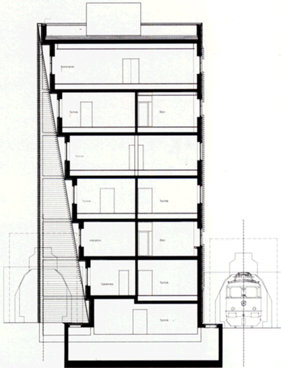
Sección transversal / Cross section
