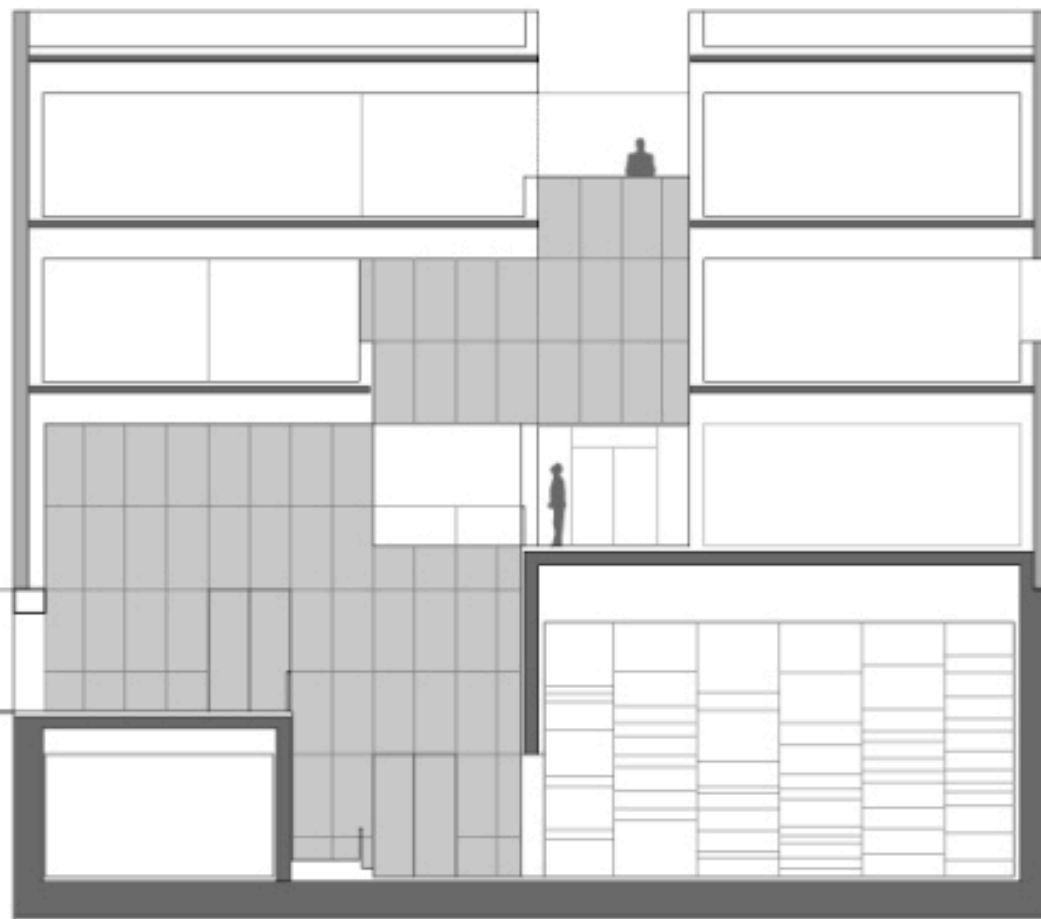
sección longitudinal e 1:200
